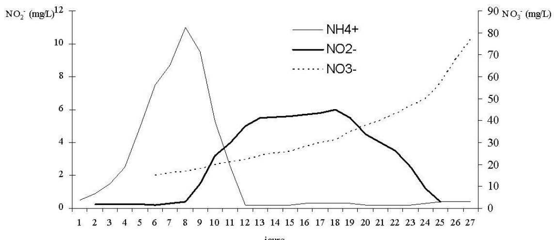
Fig. 5 : Evolution des concentrations en ammonium (NH 4 + ), nitrite (NO 2 - ) et nitrate (NO 3 - ) lors de la mise en eau d'un aquarium
